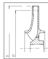
Redução do diâmetro externo do rotor para bomba centrífuga mediante torneamento.
