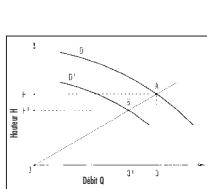
Diagramme pour déterminer le diamètre de tournage.
