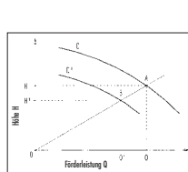
Diagramm zur Bestimmung des Drehdurchmessers.
