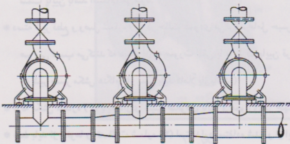
شکل ۱۰- اتصال چند پمپ به لوله کلکتور
